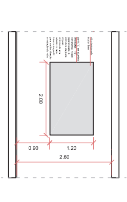
5 Vista frontal esquadria 1:75
