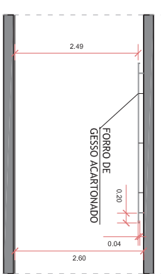
3 Corte B B' 1:75
