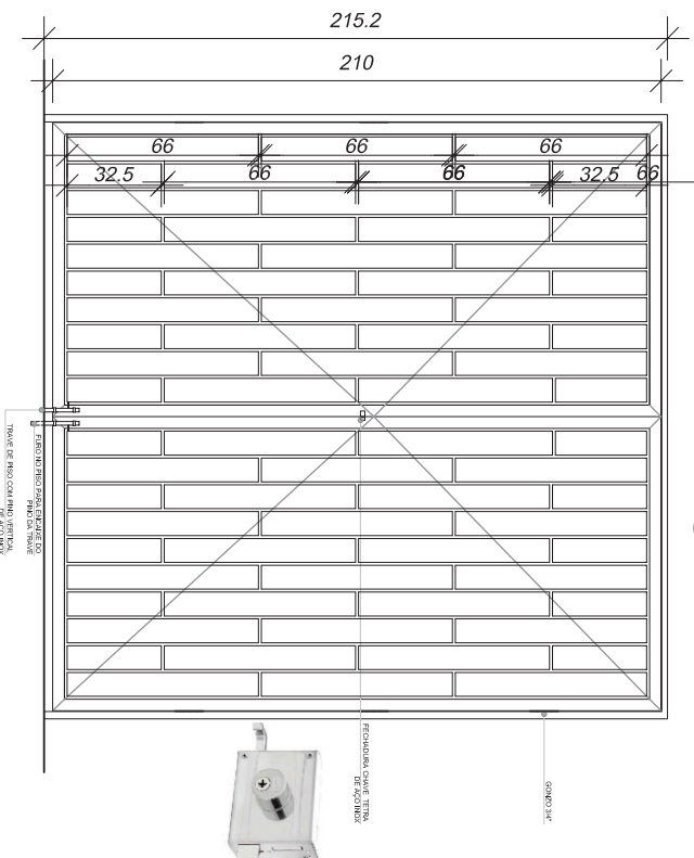
1 1:20 PLANTA BAIXA
