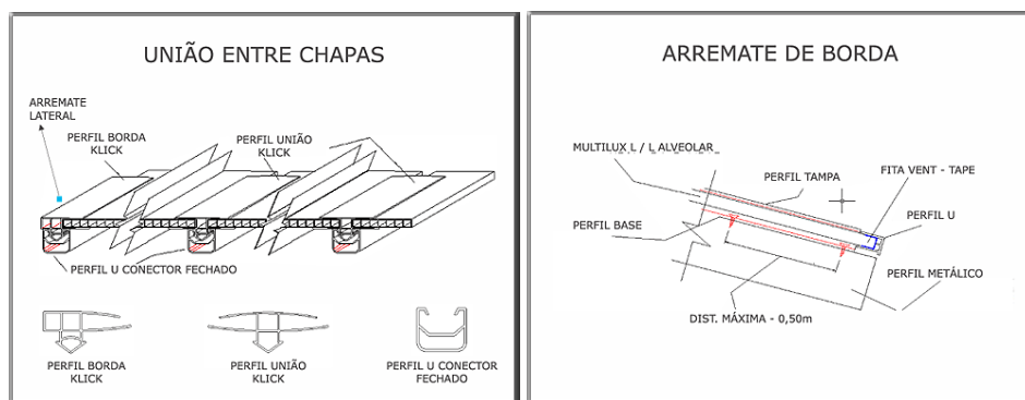
Figura 1 Sistema de cobertura com chapa alveolar, da Replaex ou Similar
