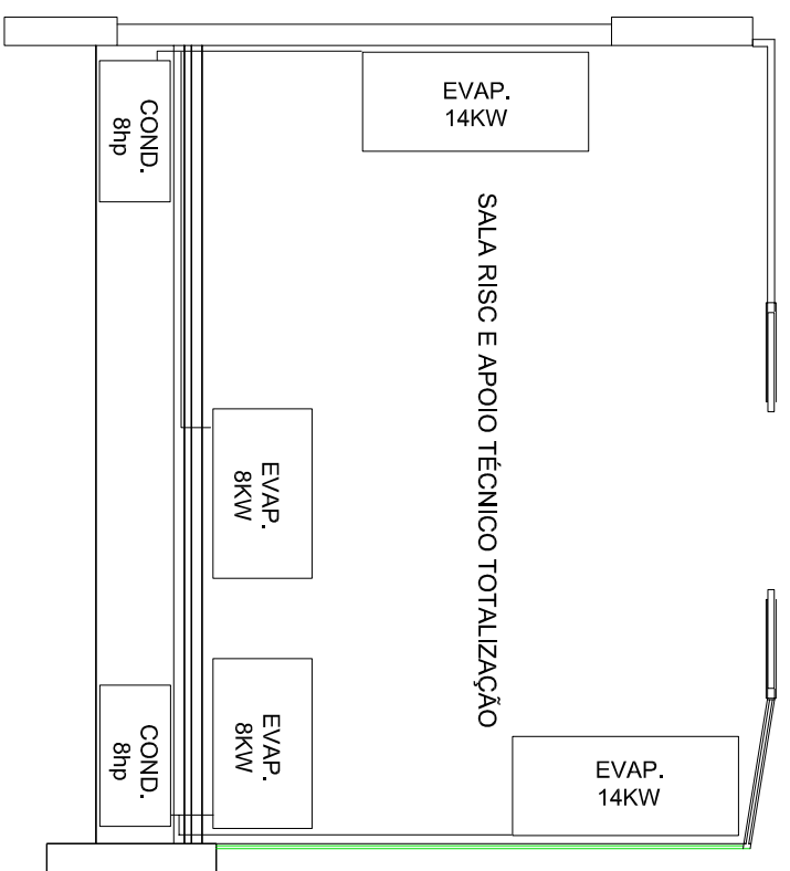
1 POSIÇÃO DOS APARELHOS DE AR CONDICIONADO SEMI ESCALA
