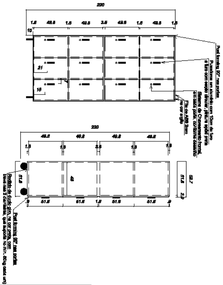
1 EROUCA 120 PLANTA BAIXA
